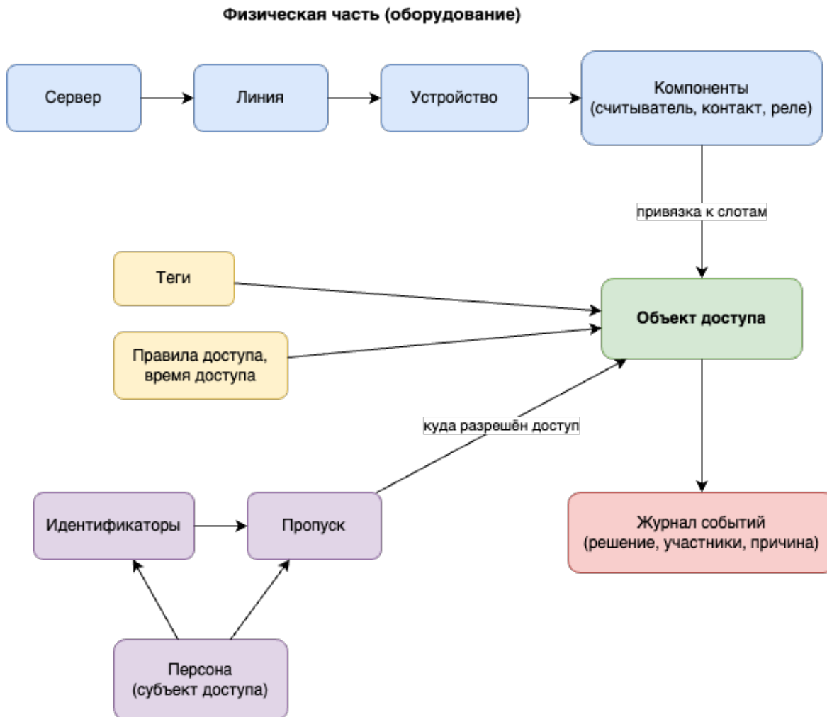
Рисунок 3.1 — Общая схема связей
